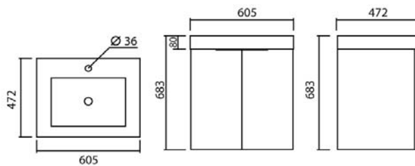
MODEL : MCN-103 (mm.)
