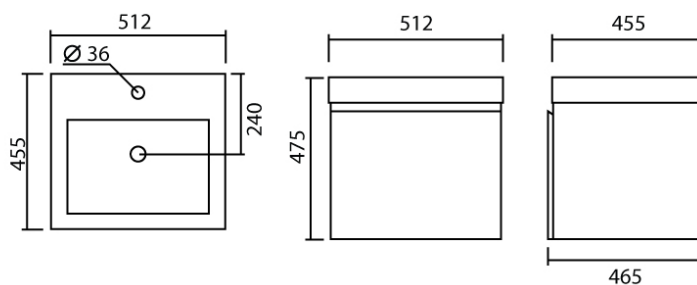
MODEL : MCN-112 (mm.)
