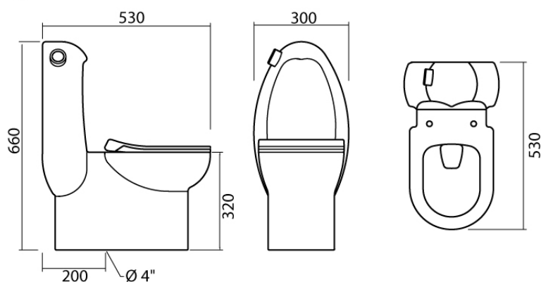
MODEL : MCP-001 (mm.)
