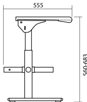
MODEL : MS304-38 (mm.)
